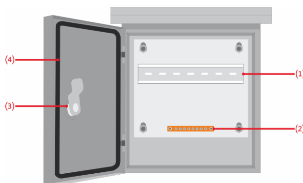
(1) DIN-рейка (2) медная шина заземления (3) защёлка (4) уплотнительное кольцо
